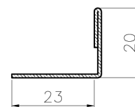
Angolare interno per profilo a "F"
