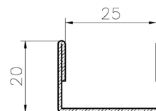
Profilo a "C"
